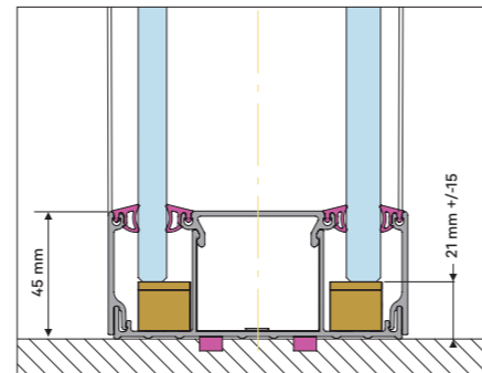
zweischalig 45 / 45 mm
