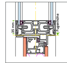
Oberer Anschlag, Drehtür Vollbau (zweischalig)
