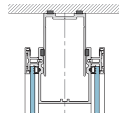
Deckenanschluss
