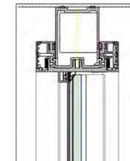
Deckenanschluss, Drehtür Glas raumhoch (einschalig)
