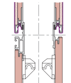
Übergang Stoff-Vollbau-Paneel
