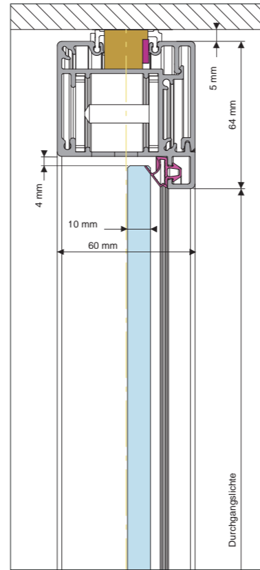
Deckenanschluss, Drehtür Glas mit Zarge, einschalig, raumhoch
