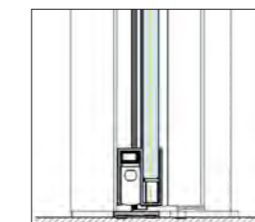
Bodenanschluss, Drehtür Glas (einschalig)
