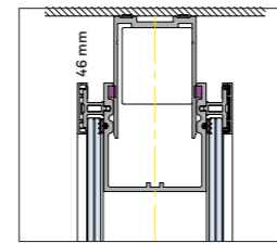
Deckenanschluss, Überbau Glas (einschalig)
