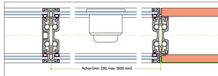
Horizontalschnitt, Elektropaneel Glas, Akustik Standard
