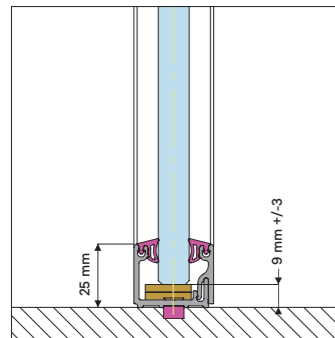
einschalig 25 / 45 mm
