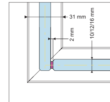
90° Verbindungen (stumpf)
