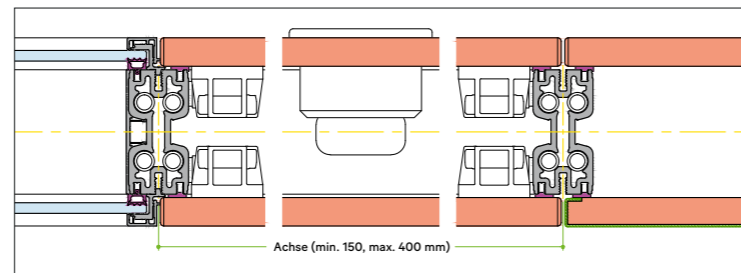
Horizontalschnitt, Elektropaneel Vollbau, Akustik Standard
