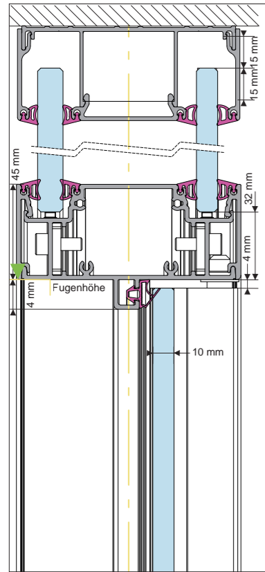
Deckenanschluss, Drehtür Glas mit Zarge, zweischalig, mit Überbau
