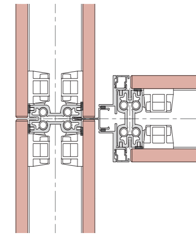
T-Knoten Smart, Anschluss an Vollbauwand
