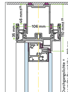
Deckenanschluss, Drehtür Glas (zweischalig)
