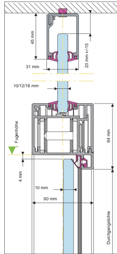
Deckenanschluss, Drehtür Glas mit Zarge, einschalig, mit Überbau
