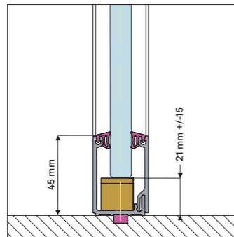
einschalig 45 / 45 mm
