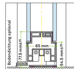
Bodenanschluss, Drehtür Glas (zweischalig)
