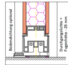
Bodenanschluss, Drehtür Vollbau (zweischalig)
