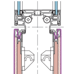
Übergang Glas-Stoff-Paneel
