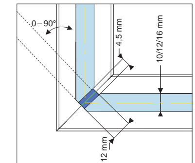
Variable 0-90° Verbindungen auf Gehung
