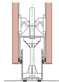
Bodenanschluss
