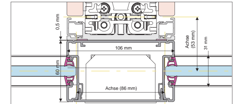
Systemtrennwand T-Anschluss an Bandraster, einschalig
