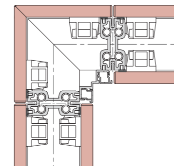
Knoten 90°, L-Verbindung in Melamin / Furnier
