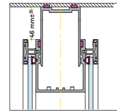
Deckenanschluss, Überbau Glas (zweischalig)
