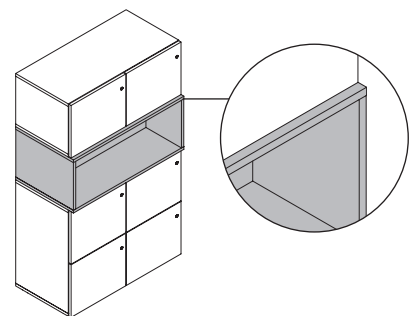
mit Überstand zu Ownly Drehtür (+21mm)
